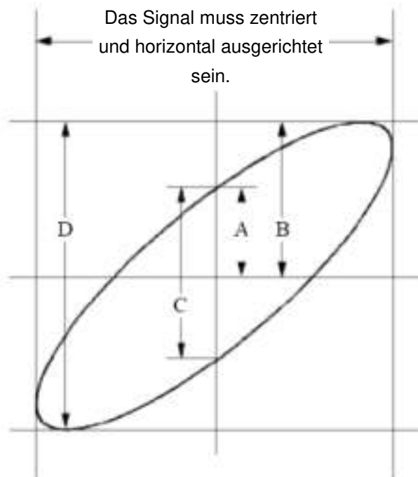
Abb. 84 Lissajous-Figur
