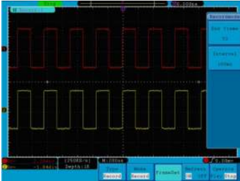
Abb. 50 Wellenform-Aufzeichnung
