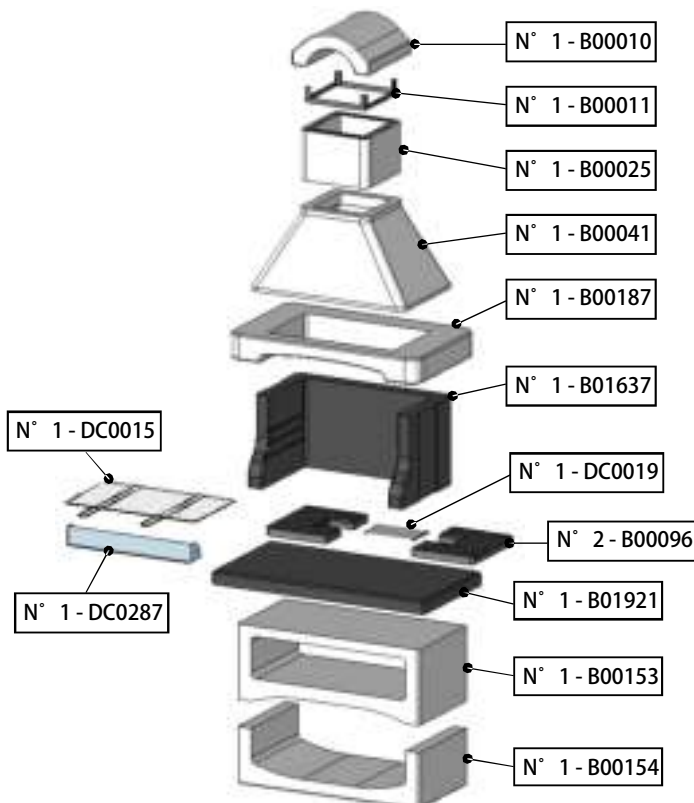
Onderdelen overzicht
