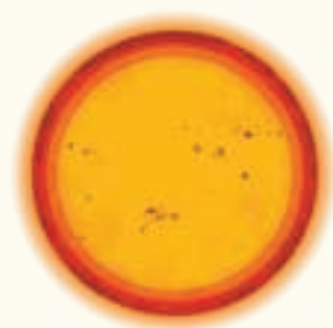
Zonnevlekken, blz. 32
