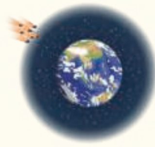
Meteorieten, blz. 10
