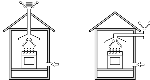
Ventilatieopening voor verbrandingslucht
