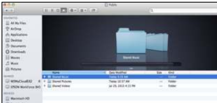
Mac Finder
