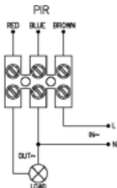
3. Bedrading van de bewegingssensor.
