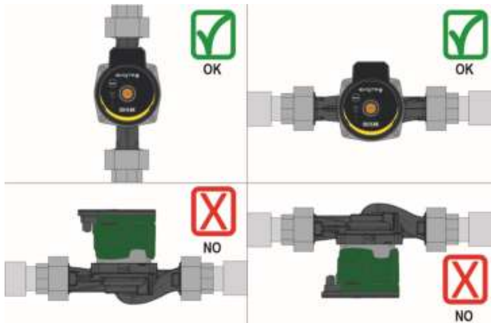
Рисунок 13: Монтажное положение
