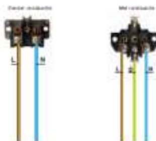
Wandcontactdoos Met/zonder randaarde
