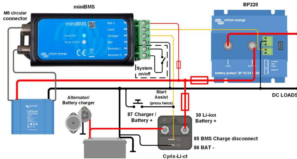
Figura 6: Esempio di applicazione per un veicolo o un natante, con interruttore on/off tra H e L (compatibile con BMS VE.Bus o miniBMS)
