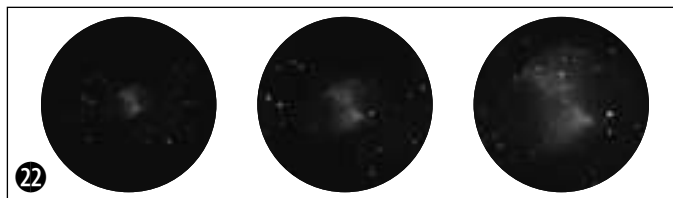
Nebulosa Manubrio nella costellazione della Volpetta (M27)
