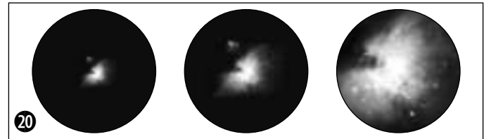
Nébuleuse d'Orion (M 42)
