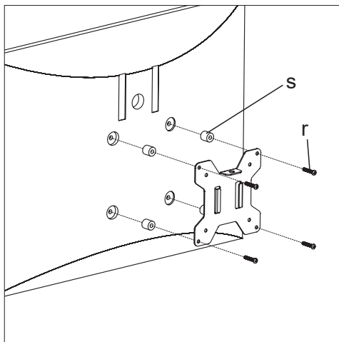
Für Monitore mit gebogener oder vertiefter Rückseite
