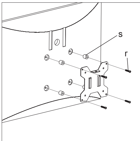
Voor monitor met gebogen of verzonken achterkant
