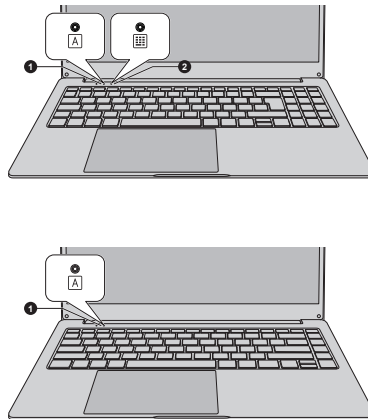
Afbeelding 4-1 Toetsenbordlampjes
