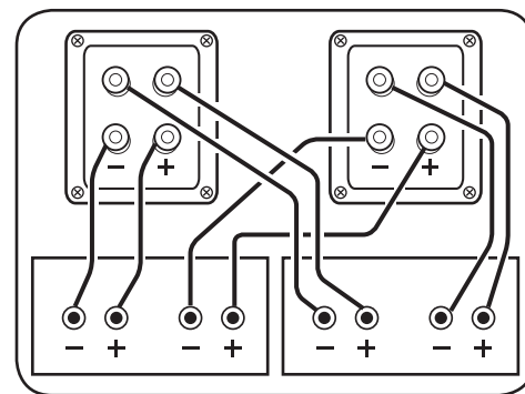
Bi-Amping
