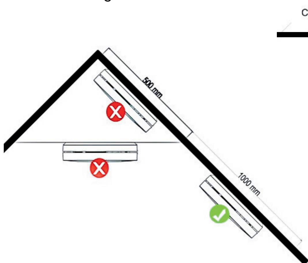
Figuur 4: Aanbevolen montage locaties
