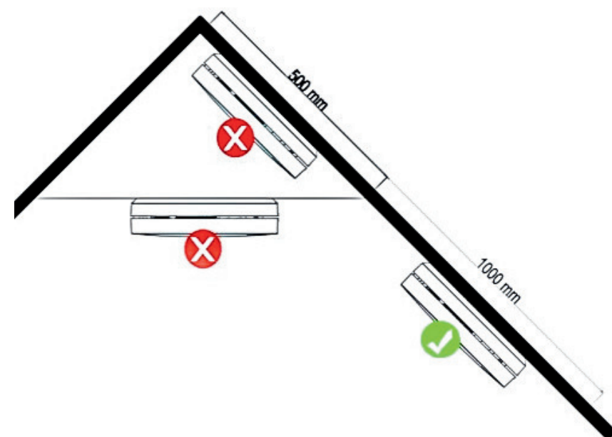
Figure 4 : Emplacements de montage recommandés
