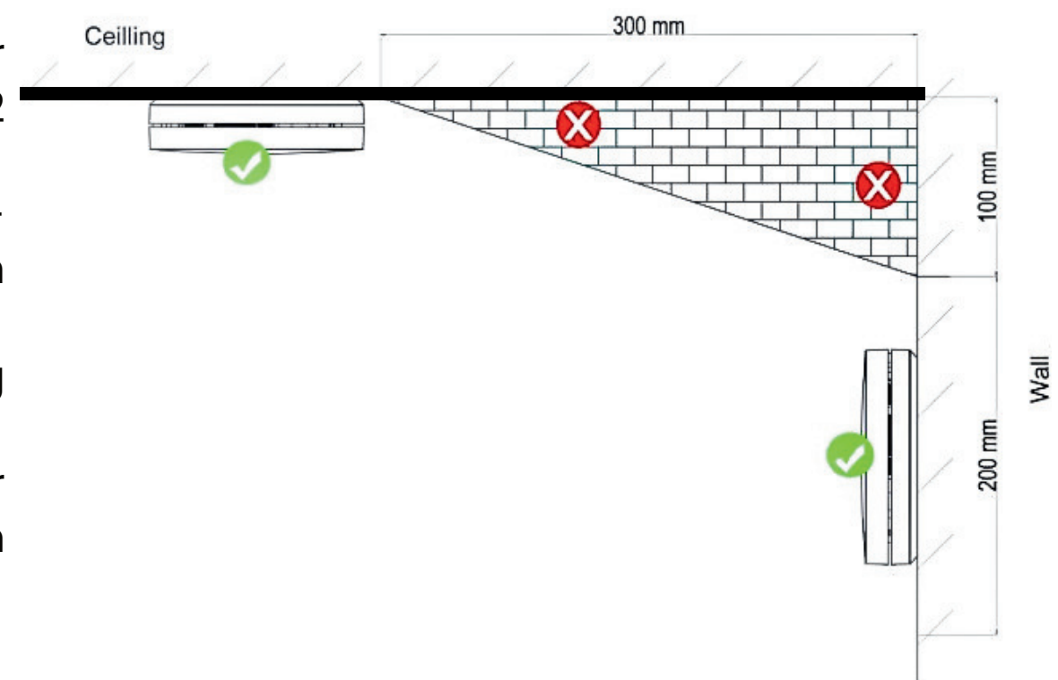
Abbildung 5: Empfohlene Montageorte
