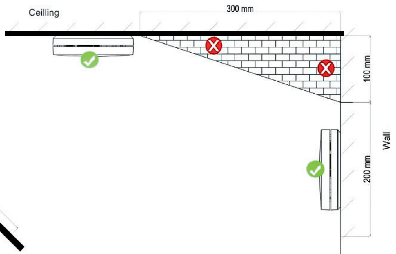
Figura 5: Ubicaciones de montaje recomendadas
