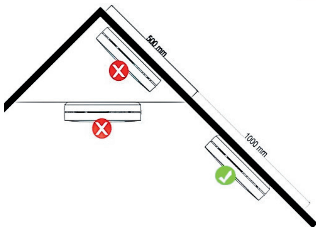
Figura 4: Ubicaciones de montaje recomendadas
