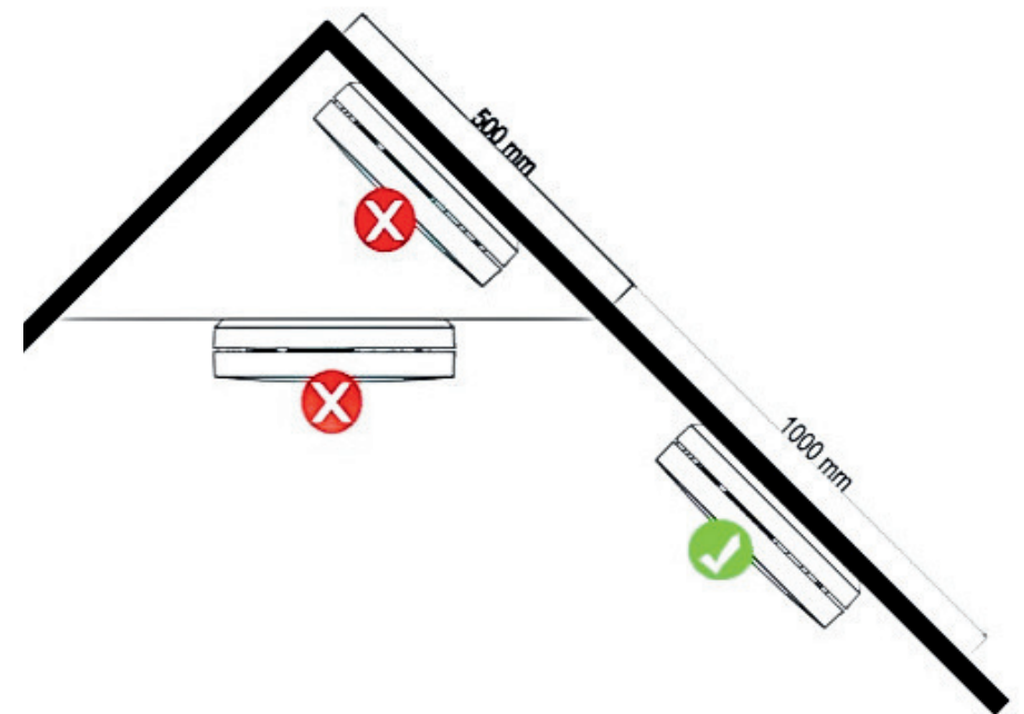
Abbildung 4: Empfohlene Montageorte
