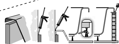
Béton cellulaire ou autre scellé au sol
