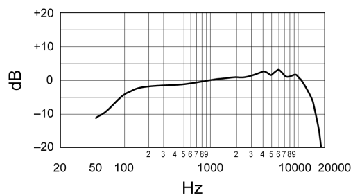
Réponse en fréquence typique
