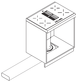
uitvoering 1, linkeruitlaat
