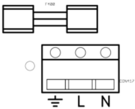
Afbeelding 2 Ingangaansluitklem
