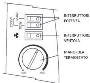
PANNELLO DI CONTROLLO
