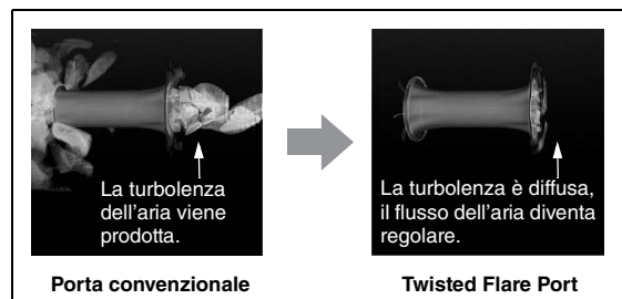
La turbolenza dell'aria in entrambe le estremità della porta crea rumore
