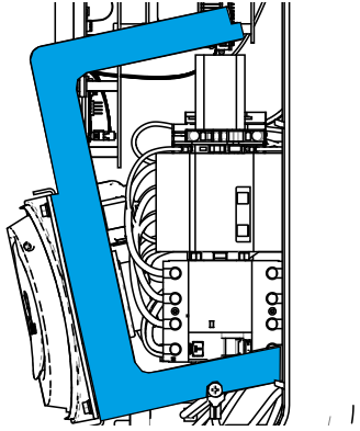
Afbeelding 5: Afneembaar subframe
