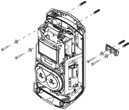
Afbeelding 3: Wandmontage
