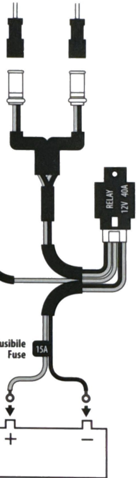
Schema di collegamento / Wiring connection Module de câblage / Esquema de conexión Verdrahtungsplan
