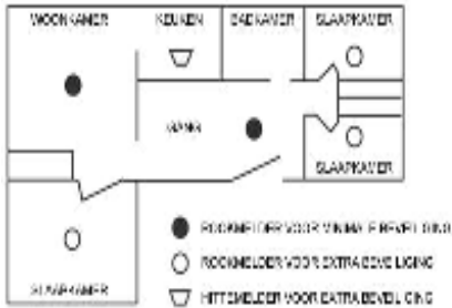
Aanbevolen locatie van rookmelders in appartementen
