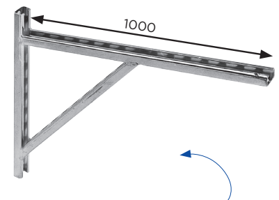
Verzinkte muurkonzole voor zware belasting verkrijgbaar per stuk
