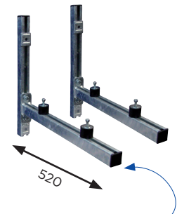
Warm verzinkte konzolen verkrijgbaar per kit
