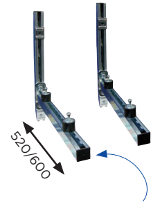
Verzinkte konzolen verkrijgbaar per kit
