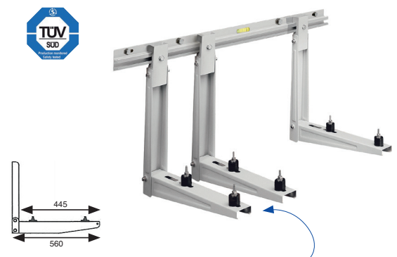
Voorzien van 3 armen voor zwaardere units
