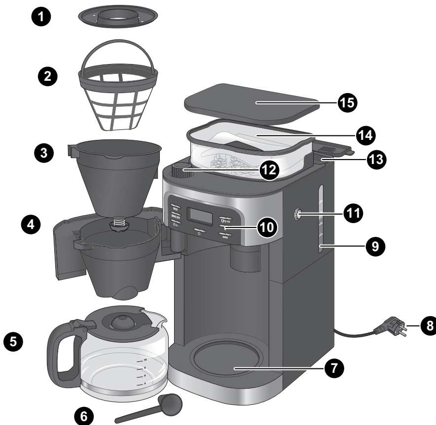
Fig. 1: Apparats dele
