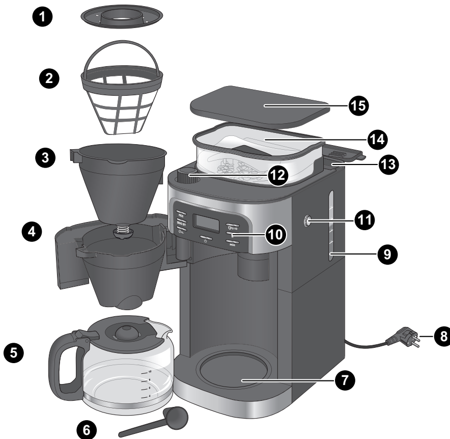
Bild 1: Apparats delar
