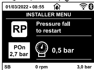
شكل 18.2: ضبط مستوى ضغط إعادة التشغيل (2)
