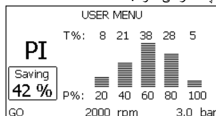
شکل 17.1: جدول نمایش مقدار توان و مدت زمان کارکرد پمپ (1)
