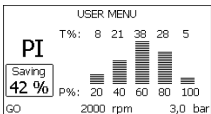
Slika 17.1: Prikaz histograma snage (1)
