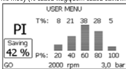
Rysunek 17.1: Wyświetlenie histogramu mocy (1)
