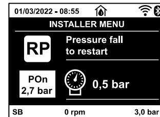
Figura 18.2: Setarea presiunii de repornire (2)
