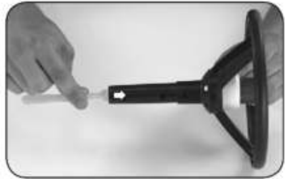
Squeeze steering clip to insert. Pressez ensemble le clip de direction pour l'insérer. Apriete la abrazadera del volante para insertarla.
