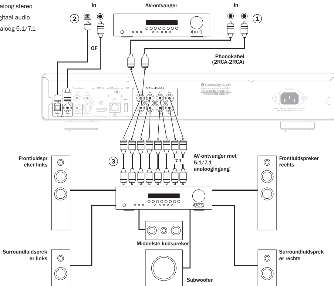
De afbeelding geeft een 5.1-kanalconfiguratie weer. Voor 7.1 twee luidsprekers achter toevoegen.
