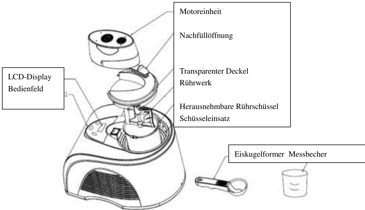
Abbildung 1 – Explosionszeichnung
