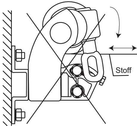
Falsche Ausführung
