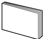
Snelstartgids
