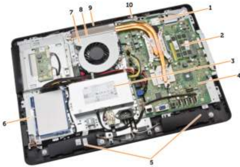
Afbeelding 2. Binnenaanzicht – 2
