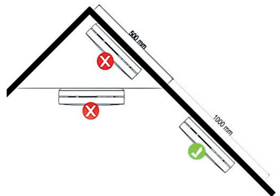
Abbildung 4: Empfohlene Montageorte
