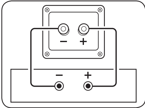
Standardanschluss
