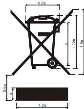
WEEE标志, 请严格按照此比例来制作 在印刷件上显示高度大于7MM(等比例缩放)
