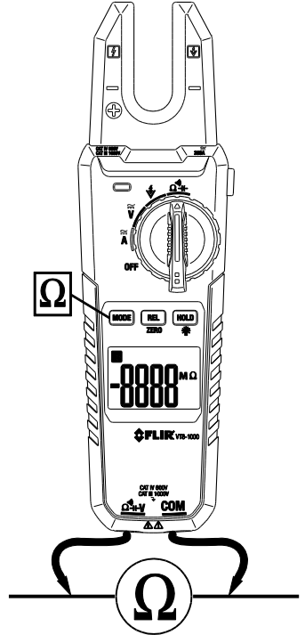
Fig. 5-4 WEERSTANDSMETINGEN
