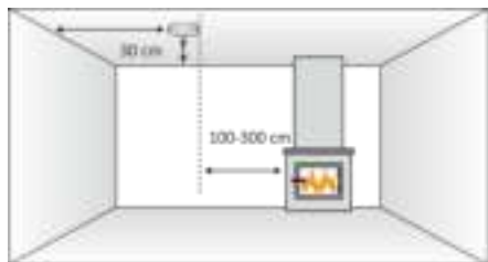
Plafond montage
