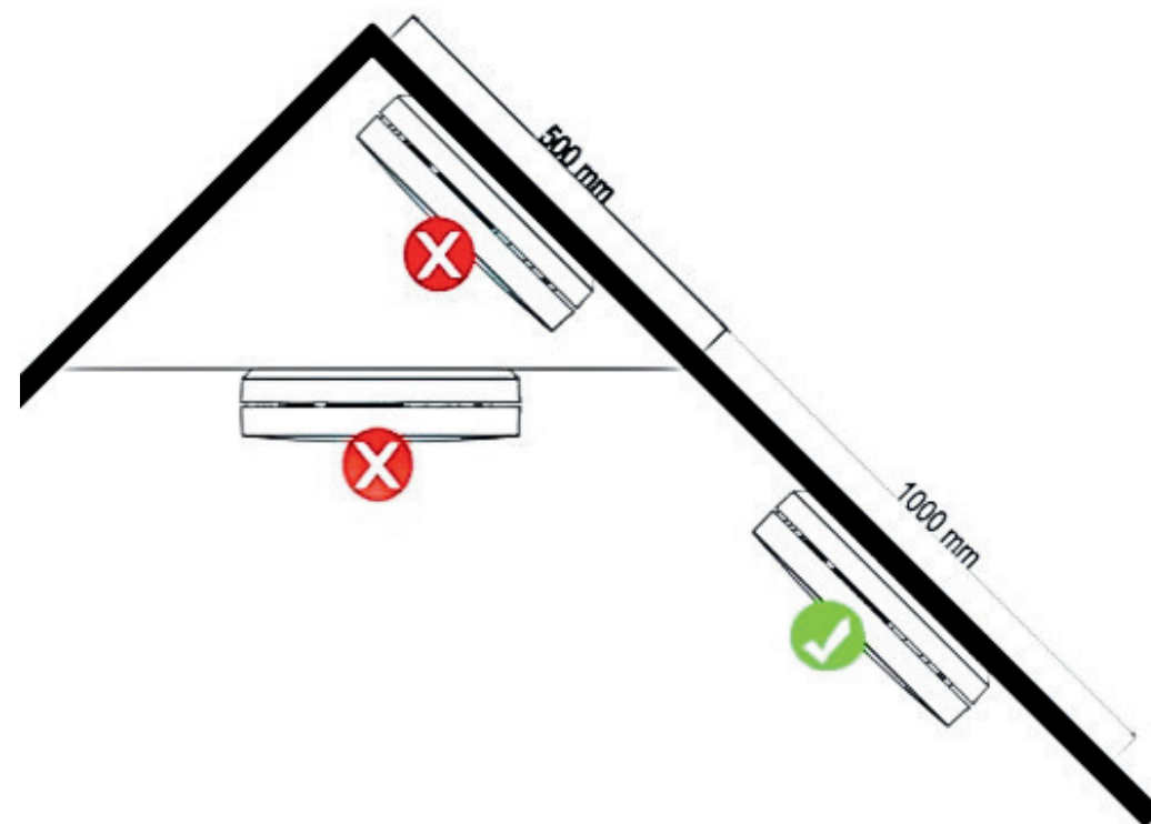
Figura 2: posizioni di montaggio consigliate
