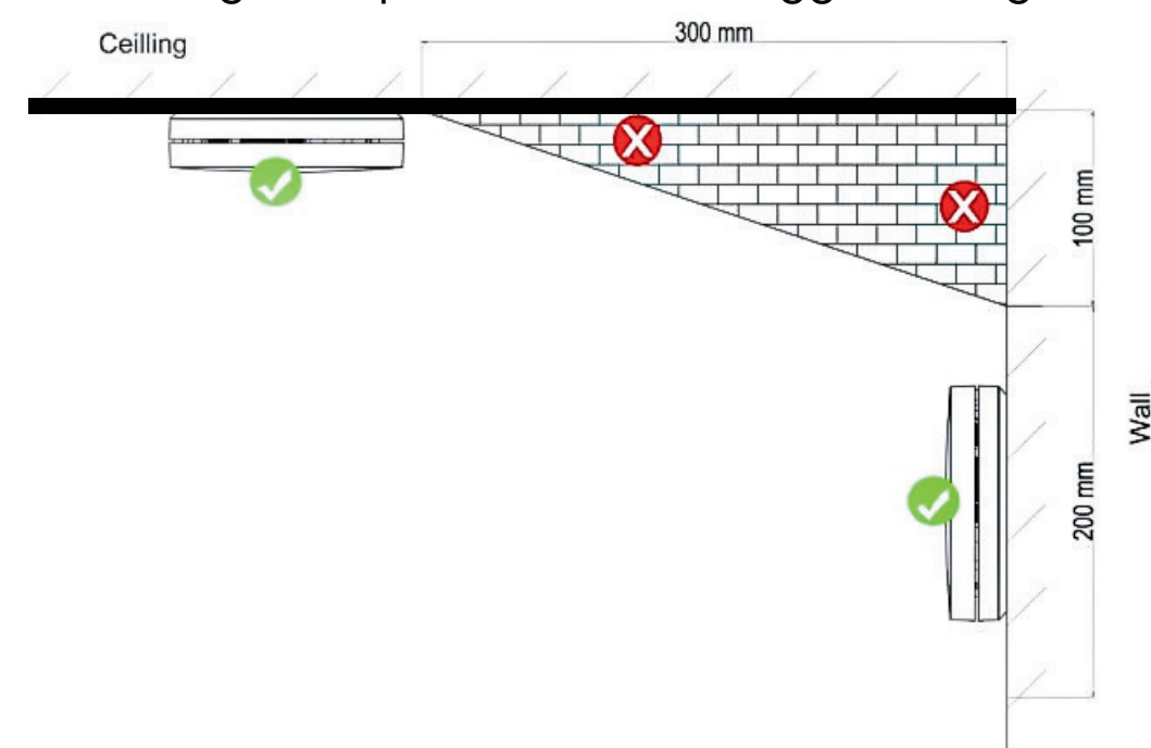
Figura 2: posizioni di montaggio consigliate
