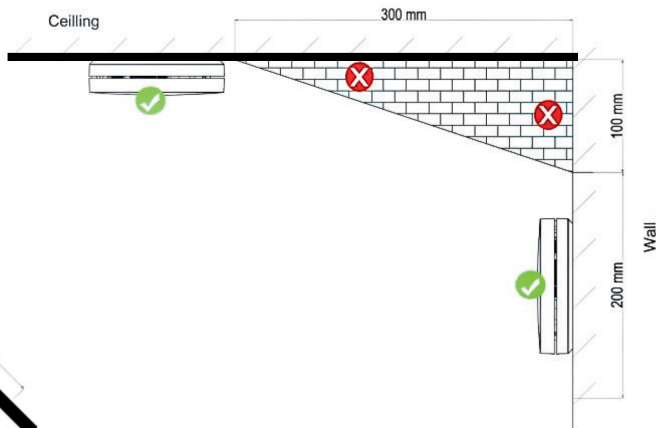
Figure 3: Emplacements de montage recommandés
