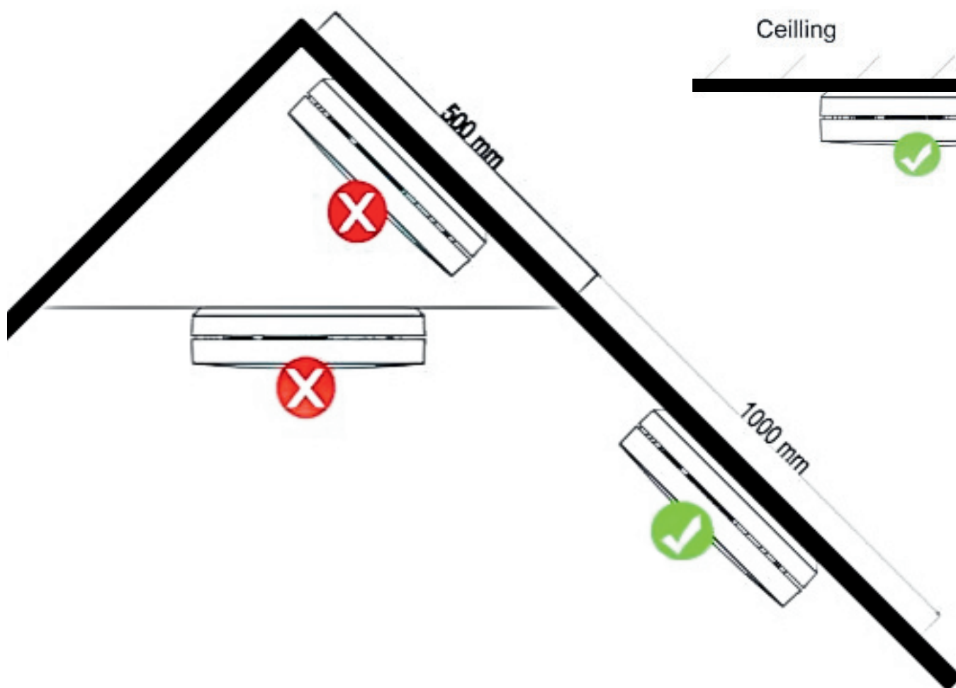
Abbildung 2: Empfohlene Montageorte
