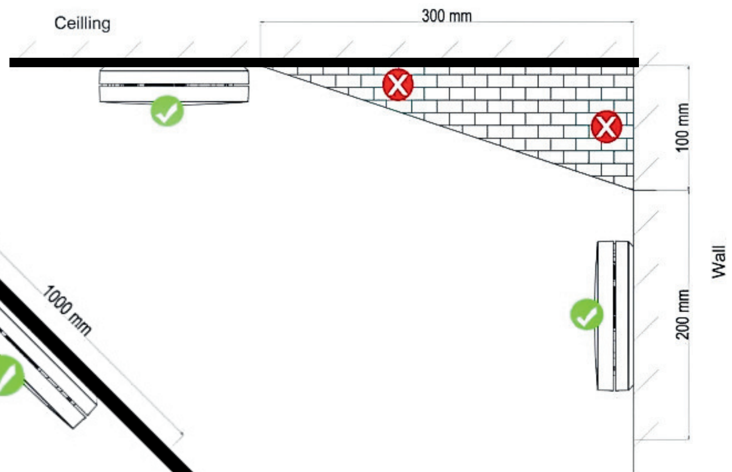
Abbildung 3: Empfohlene Montageorte
