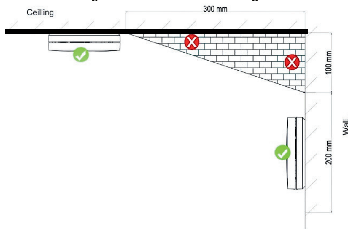
Figuur 3: Aanbevolen montagelocaties
