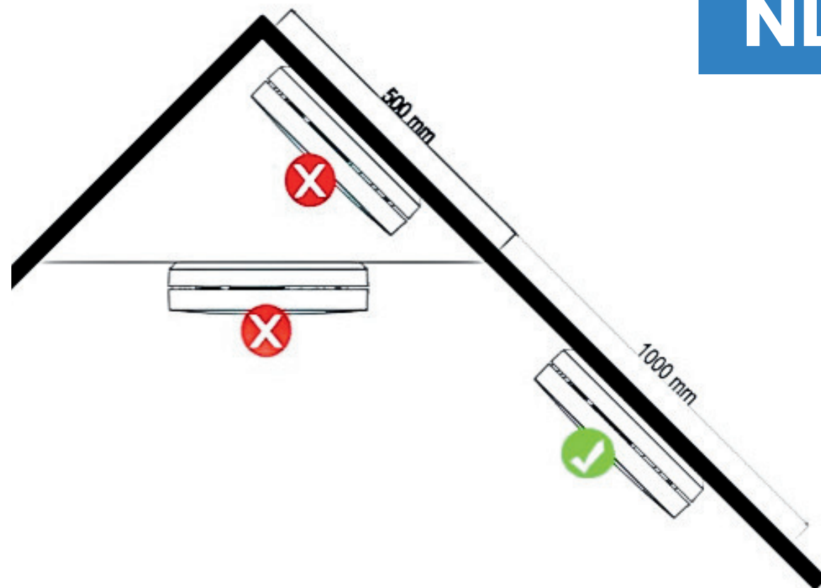
Figuur 2: Aanbevolen montagelocaties
