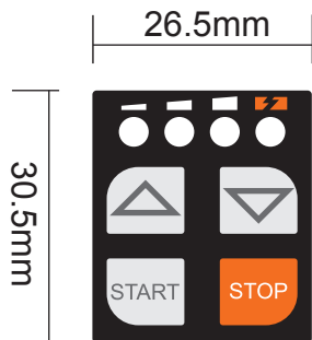
薄膜开关，四圆孔镂空
