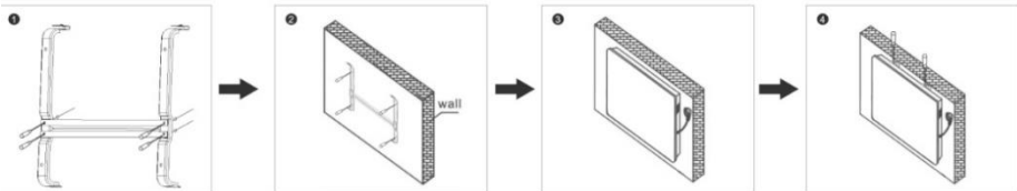
Abb. 2 Wandmontage
