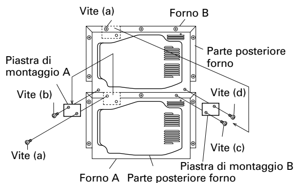
Figura A. Modo di fissare i due forni.
