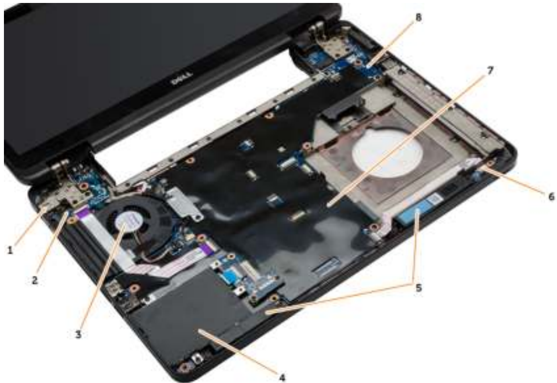
Afbeelding 2. Binnenaanzicht – voorzijde
