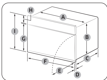
Uuni (mm)
