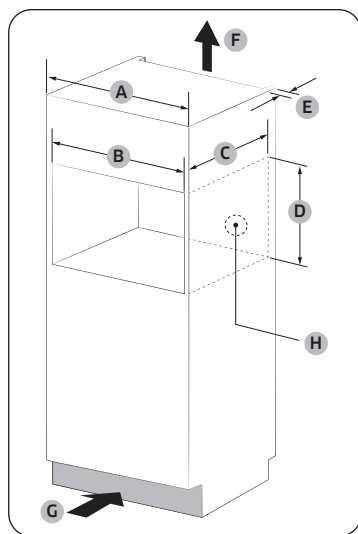
Inbouwkast (mm)
