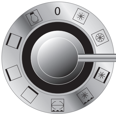
Funktionsshalter : Elektrischer Öfen mit einer breite von 60 und 80 cm
