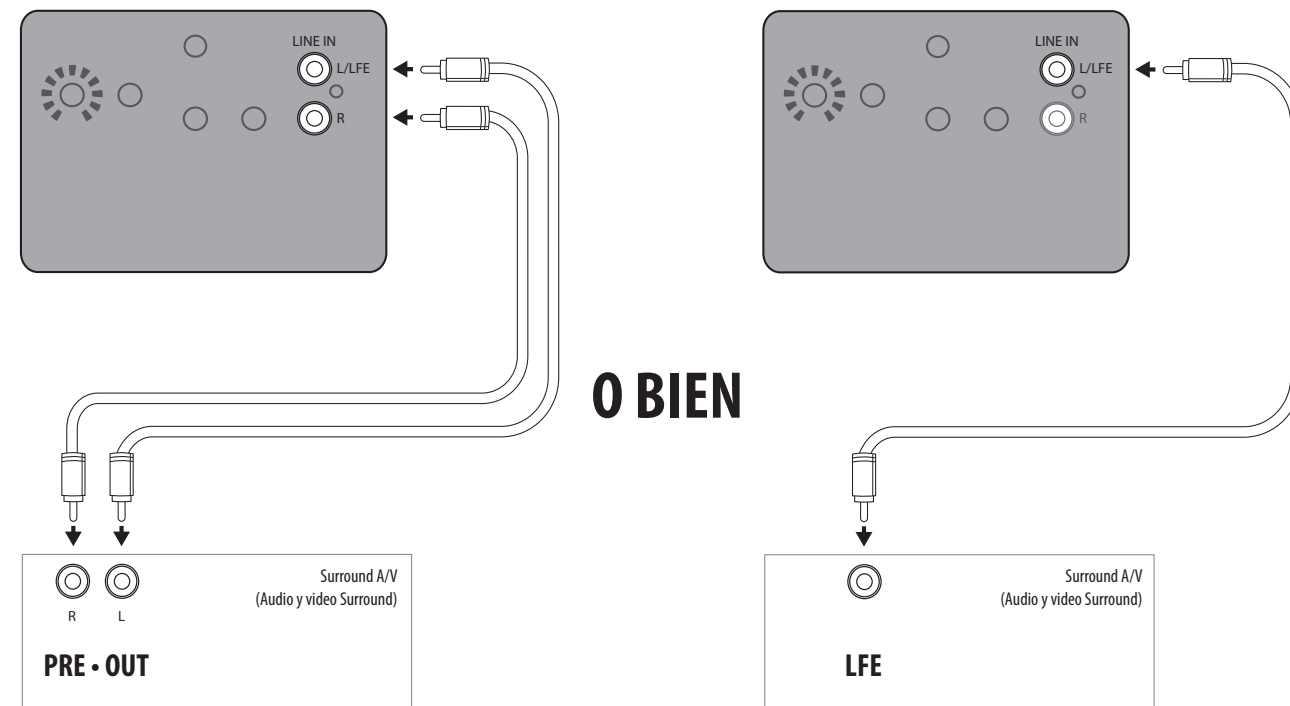
Figura 2 Cableado De Los Subwoofers J 110, J 112
