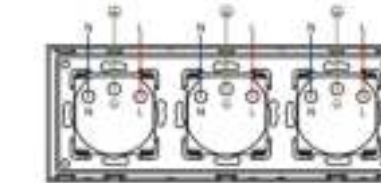
Aansluitschema van een drievoudig stopcontact (I)
