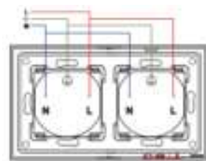
Aansluitschema van een tweevoudig stopcontact (II)
