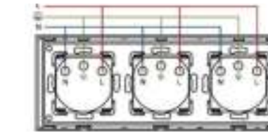
Aansluitschema van een drievoudig stopcontact (II)
