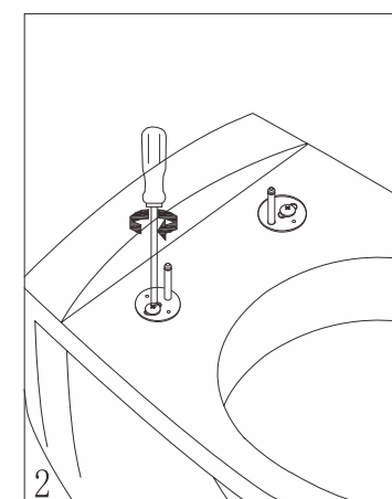
2 Draai de schroeven vast
