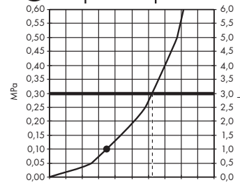
Q = l/min 0 3 6 9 12 15 18 21 24 27 30 Q = l/sec 0 0,1 0,2 0,3 0,4 0,5 Croma 220 Air 1jet 26464000
