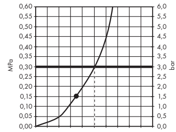
Q = l/min 0 3 6 9 12 15 18 21 24 27 30 Q = l/sec 0 0,1 0,2 0,3 0,4 0,5 Croma 280 Air 1jet 26220000
