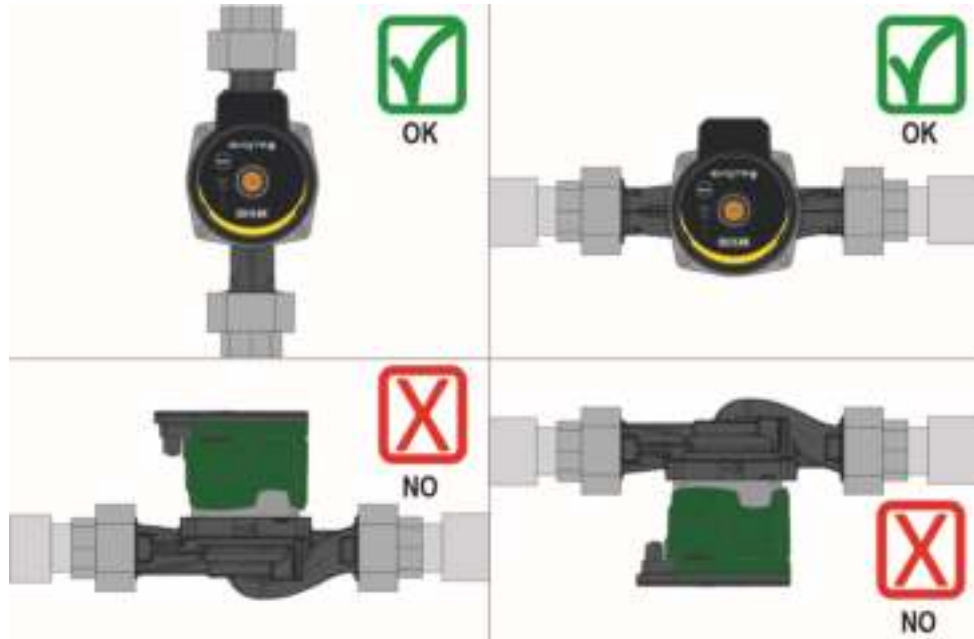
Kuva 13: Asennusasento
