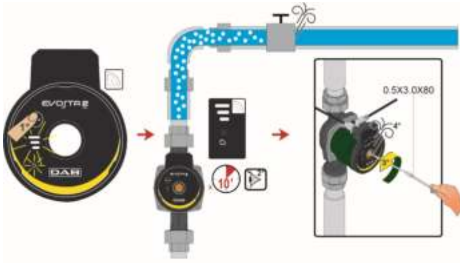
Kuva 17: Pumpun ilmaus
