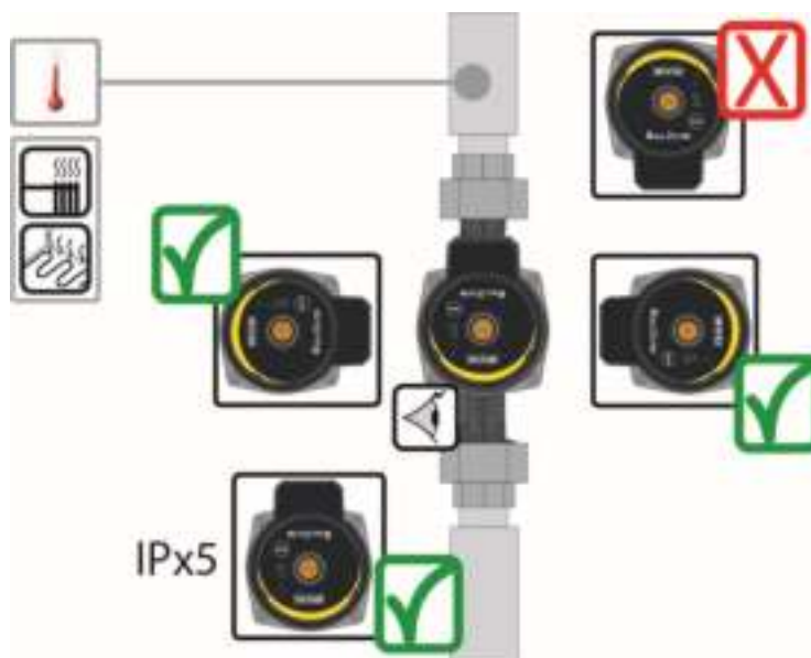
Fig 14: Användargränssnittets positioner
