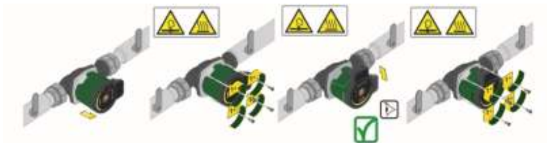
Image 15: Changement de position de l'interface utilisateur
