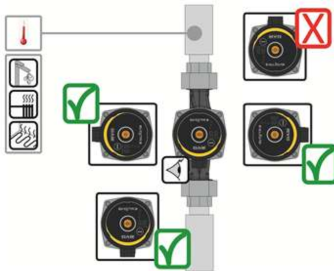
Kuva 4: Käyttöliittymän asennot
