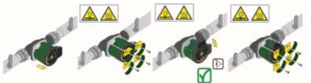
Figura 15: Troca de posição da interface utilizador
