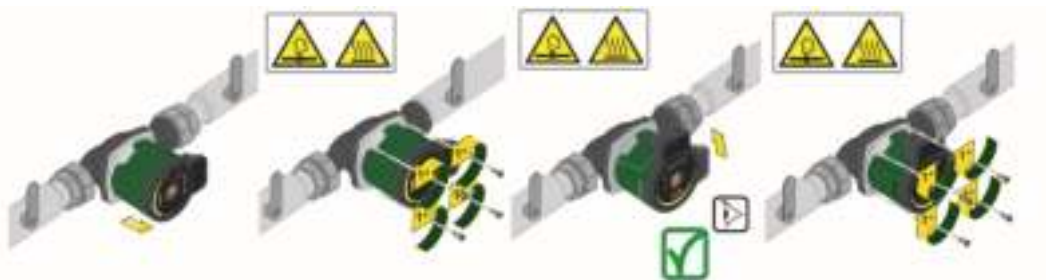
Figura 15: Cambiamento della posizione dell'interfaccia utente
