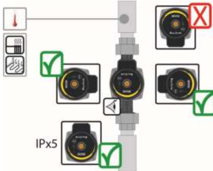
Kuva 14: Käyttöliittymän asennot
