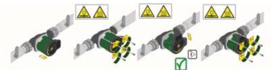
Obrázek 15: Změna polohy uživatelského rozhraní
