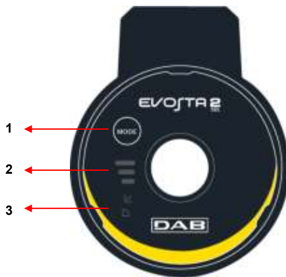
Fig. 18: Display
