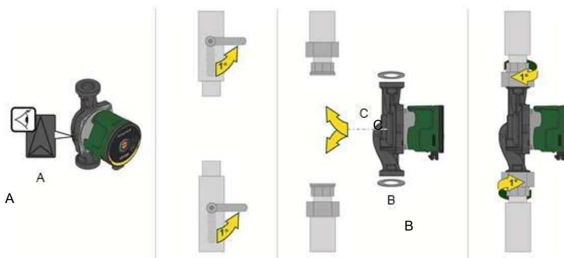
Рисунок 2: Монтаж EVOSTA2, EVOSTA3
