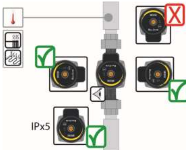
Fig. 14: Brugergænsefladens positioner
