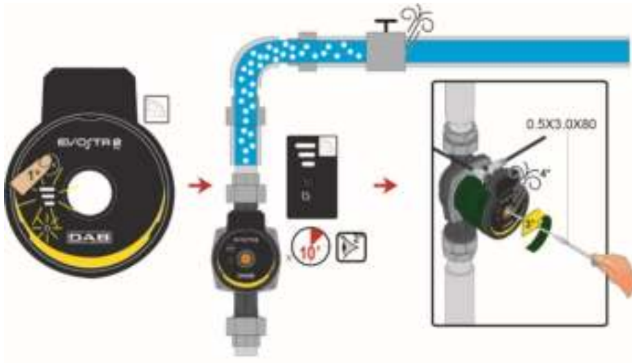
17. ábra: Pumpa légtüresztés
