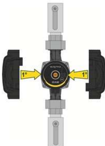
Rysunek 7: Izolacja korpusu pompy
