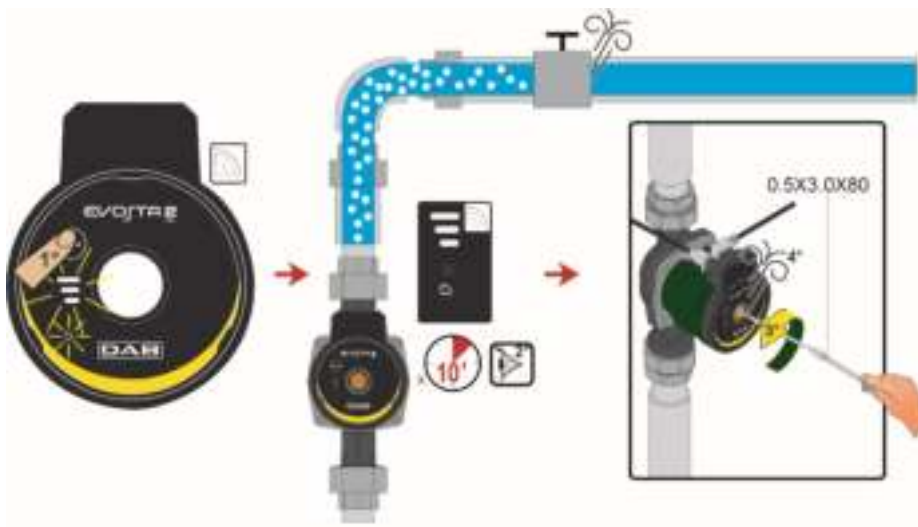
Figura 17: Aerisirea pompei
