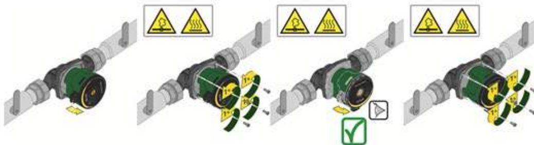
Фигура 6: Промяна на позицията на потребителския интерфейс
