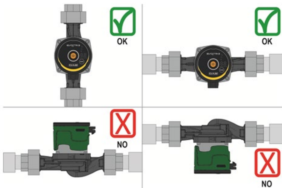
Obrázek.3: Poloha montáže
