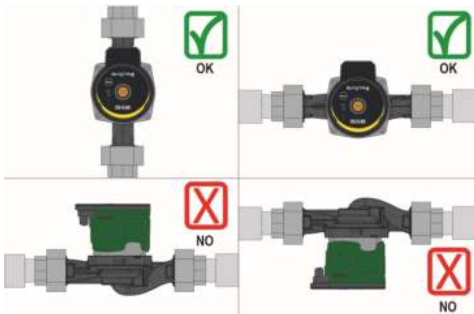
13. ábra:Szerelési pozíció
