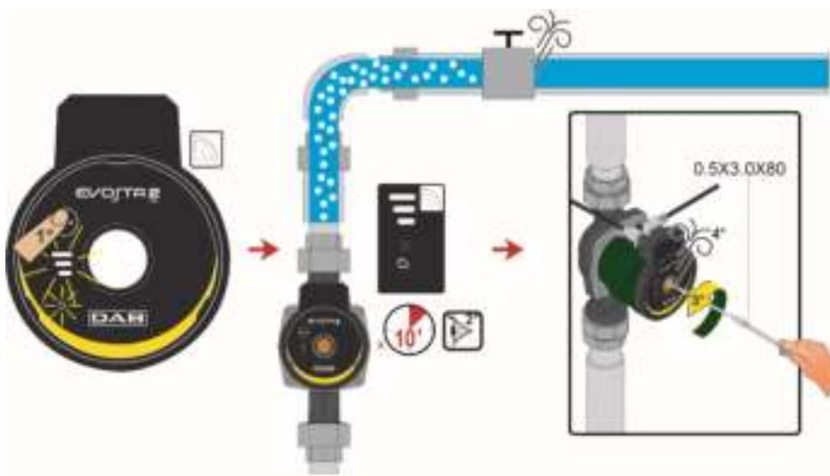
Obrázok 17: Odvzdušnenie čerpadla
