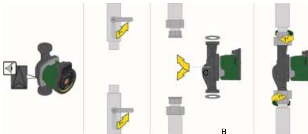
Фигура 12: Монтиране на EVOSTA2 SOL
