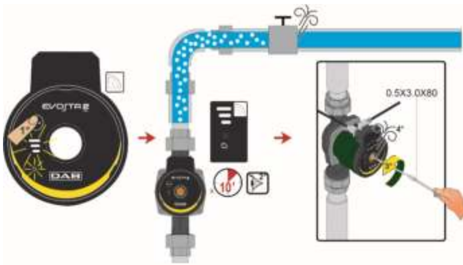
Obrázek 17: Odvzdušnění čerpadla
