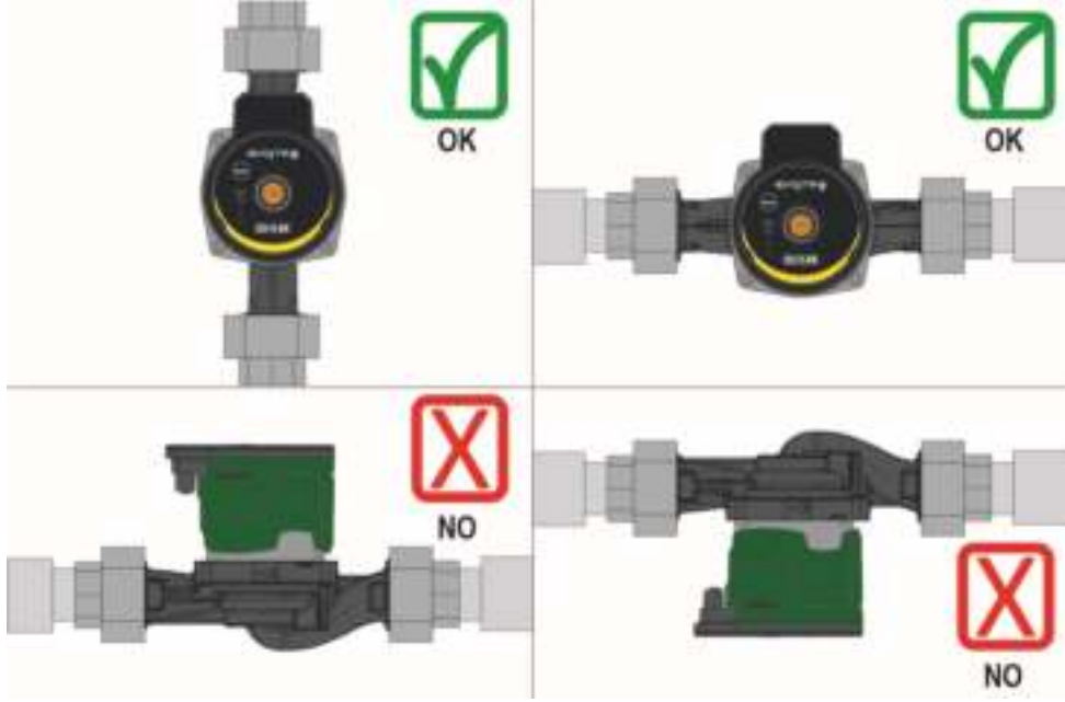
Resim 13: Montaj pozisyonu
