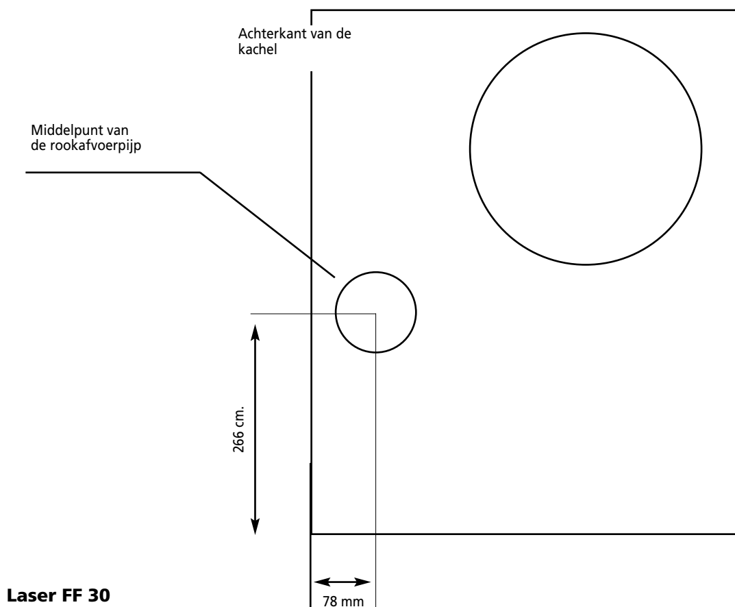
Afb. 1-3 Boorsjabloon
